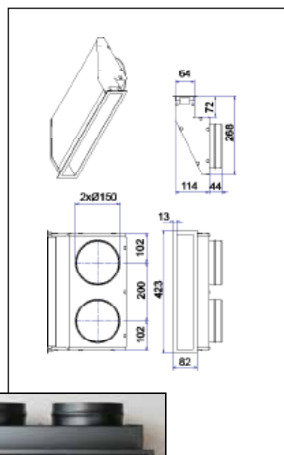
Designrooster ( uitlaat ) met 2 aansluitingen /
