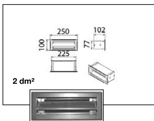
Aanzuigrooster ( inlaat )
