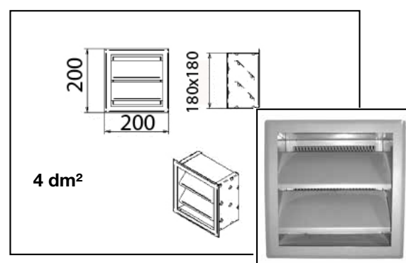
Aanzuigrooster (inlaat)
