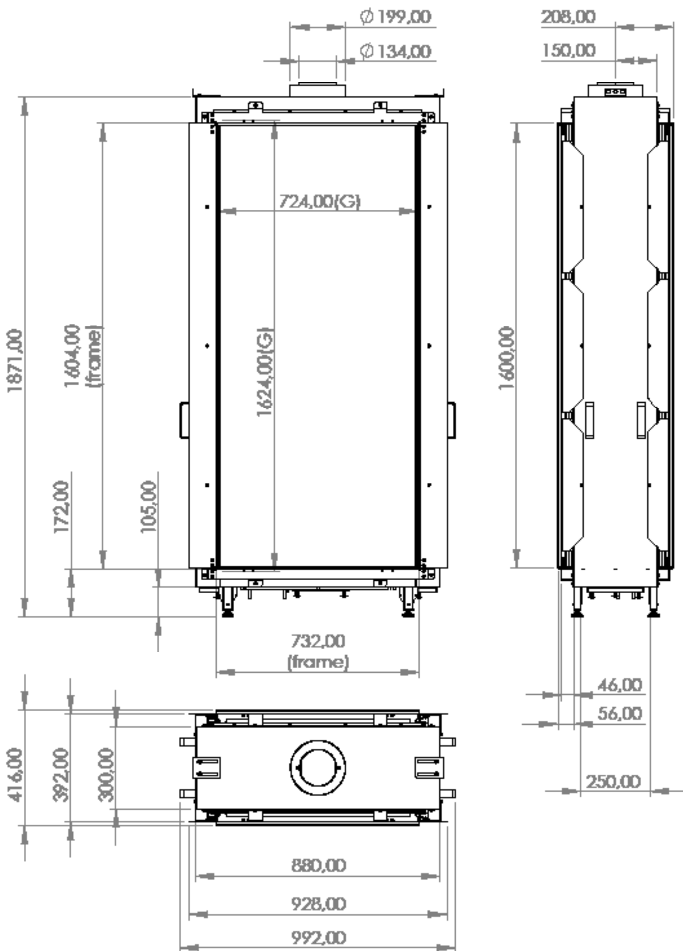
Afbeelding I.A Maattekening van de Sky L T
